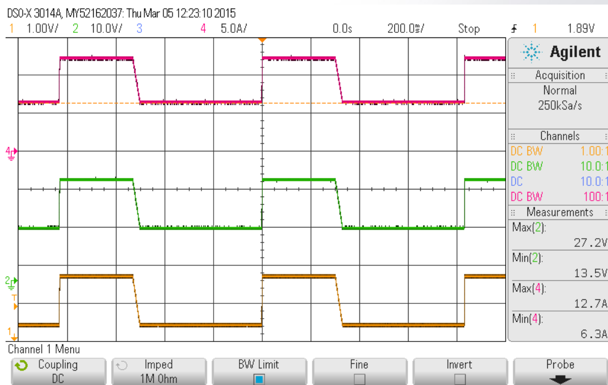
Abbildung 2: CH1= U_{in} ; CH2= U_{out} ; CH4= I_{out}
