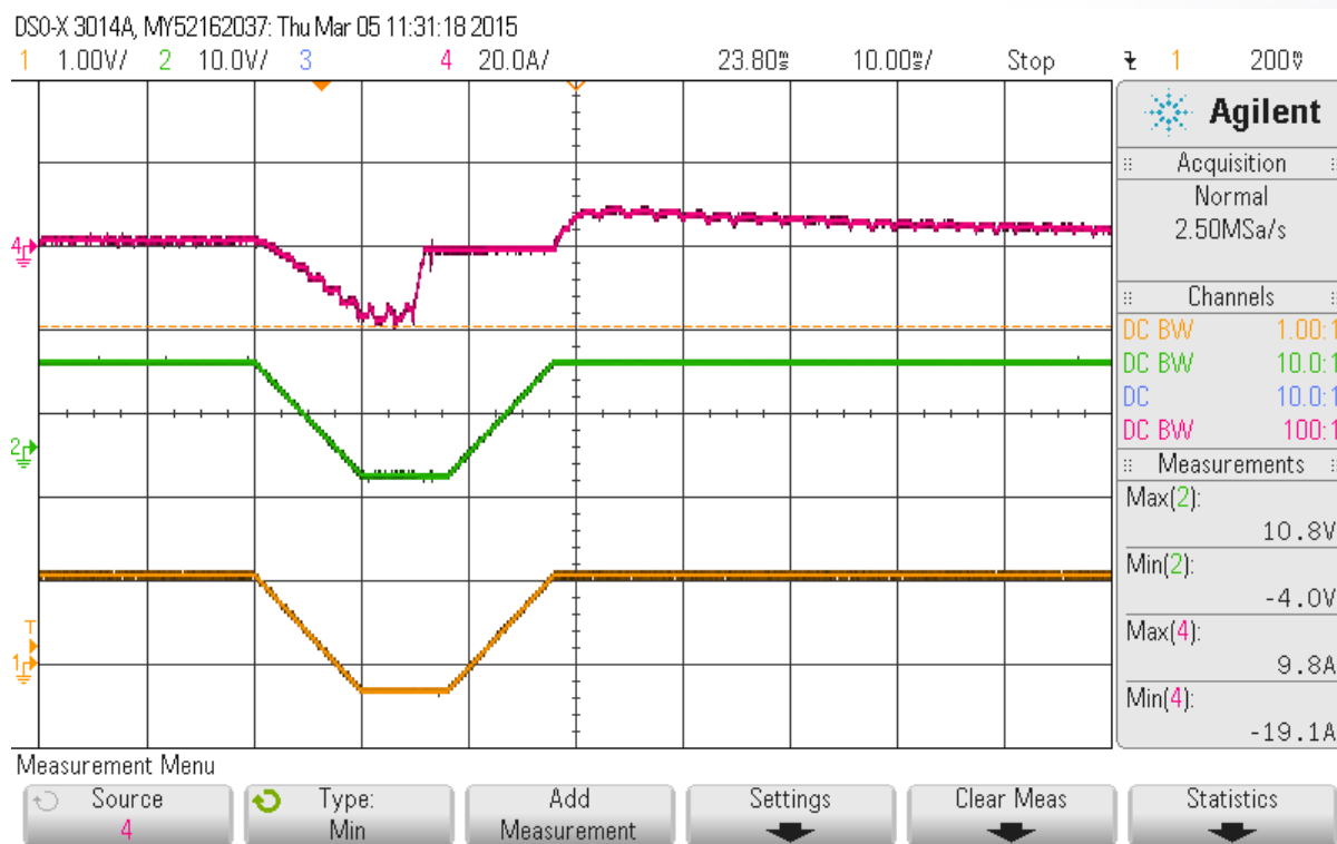
Abbildung 10: CH1=Uin; CH2=Uout;CH4=Iout
