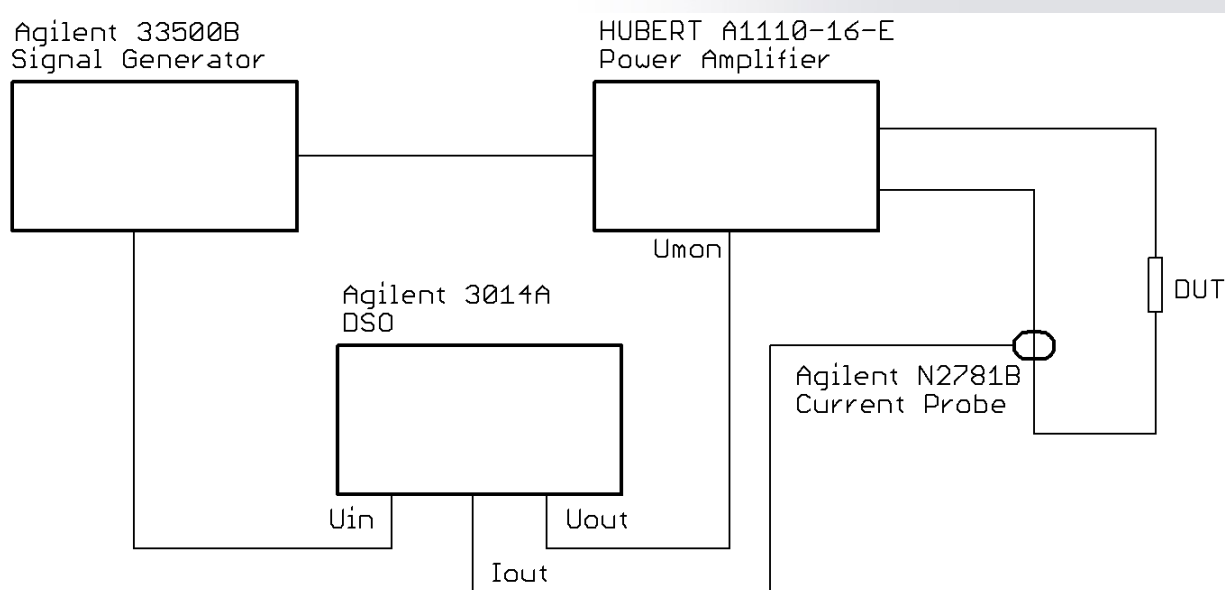
Abbildung 1: Test Setup
