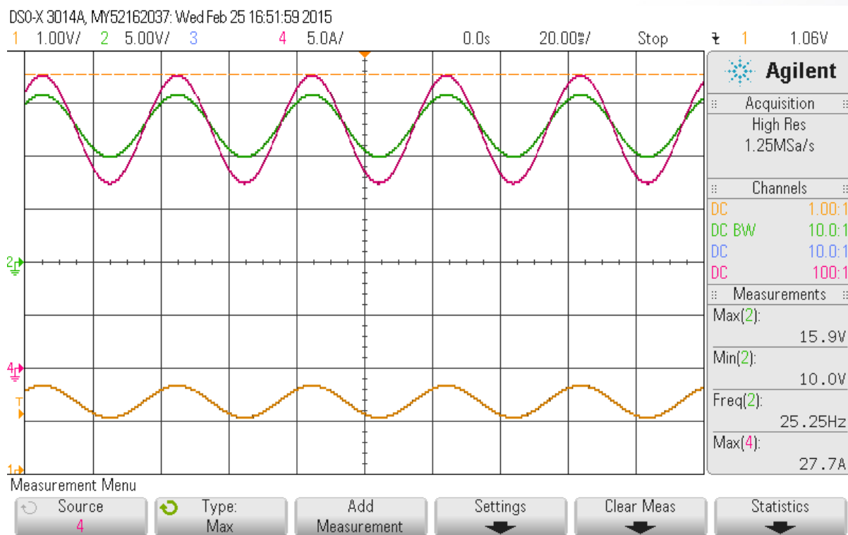
Abbildung 4: CH1=U in ; CH2=U out ;CH4=I out ; f=25 Hz
