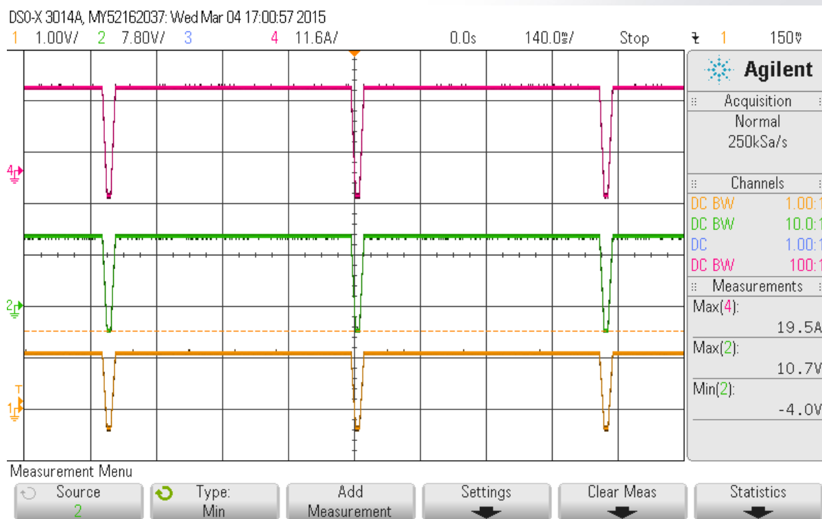
Abbildung 9: CH1= U_{in} ; CH2= U_{out} ; CH4= I_{out}
