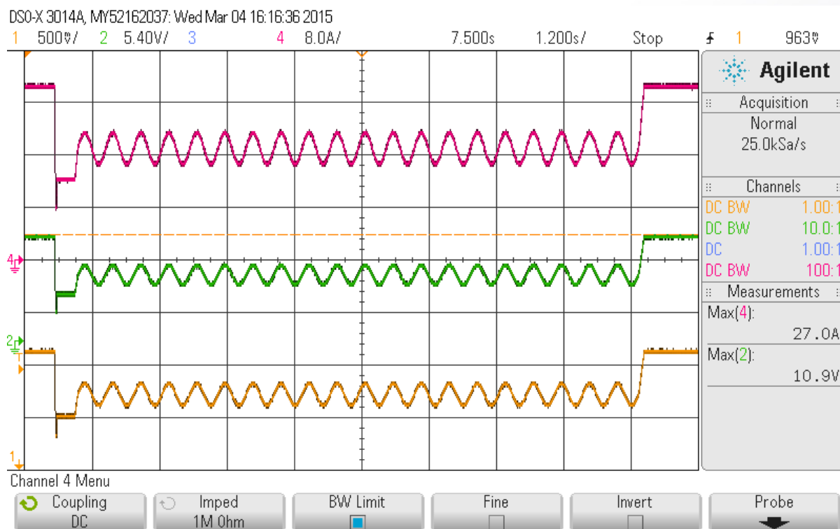
Abbildung 7: CH1=Uin; CH2=Uout;CH4=Iout
