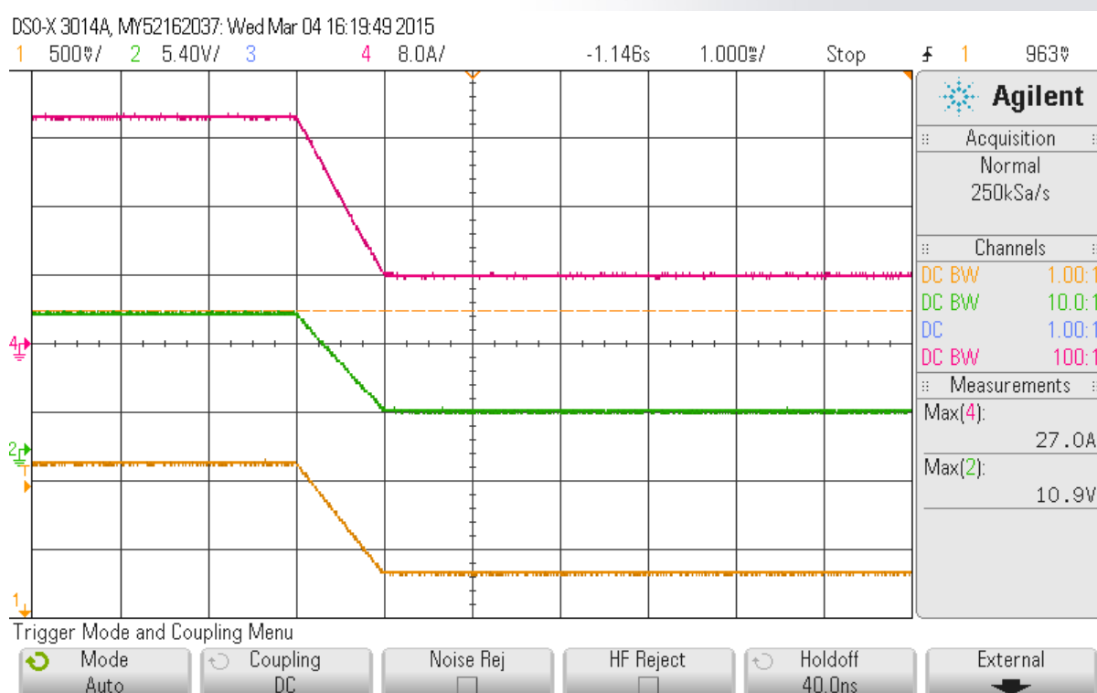
Abbildung 8: CH1=Uin; CH2=Uout;CH4=Iout
