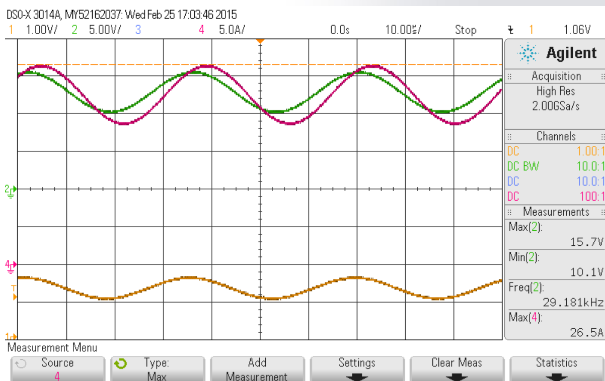
Abbildung 5: CH1=U in ; CH2=U out ;CH4=I out , f=29 kHz
