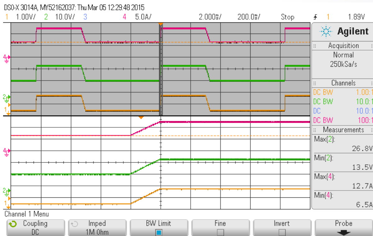
Abbildung 3: CH1=Uin; CH2=Uout;CH4=Iout
